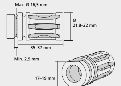
NATO A1/A2 -liekinsamuttimien mitoitus QM2-kiinnitykselle.
